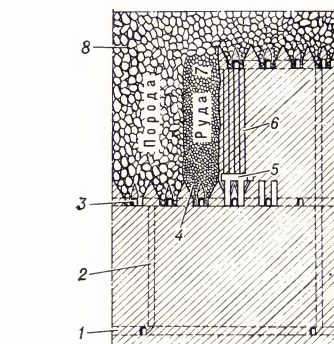
Рис. 6. Одностадийный вариант системы подэтажного обрушения с отбойкой руды вертикальным слоем в зажатой среде: 1 — выработки откаточного горизонта; 2 — рудоспуск; 3 — подэтажные выработки; 4 — выпускные воронки; 5 — буровые выработки; 6 — скважины; 7 — отбитая руда; 8 — обрушенная порода.
